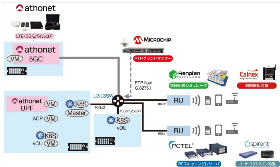
【図 1：丸文ローカル 5G の構成図】
