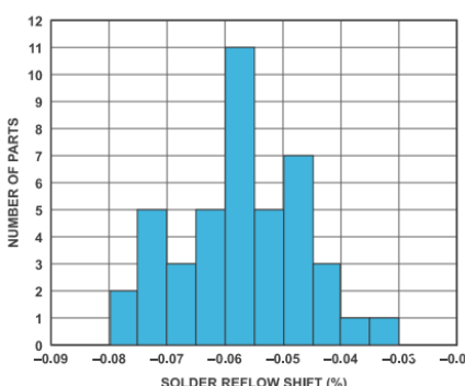
リフローはんだ熱による電圧シフト
