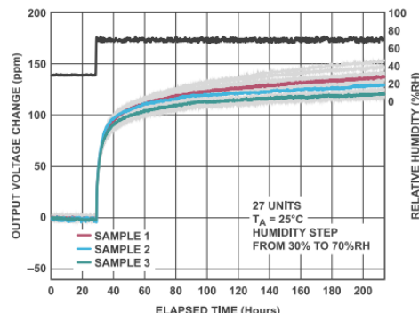
湿度による電圧変動
