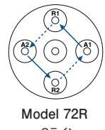
Model 72R 2ライン リバーススイッチ
