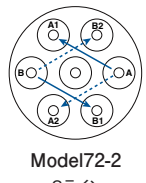
Model 72-2 2ライン 2回路へ接続可能
