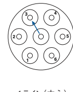
1ライン(中心) 6回路へ接続可能
