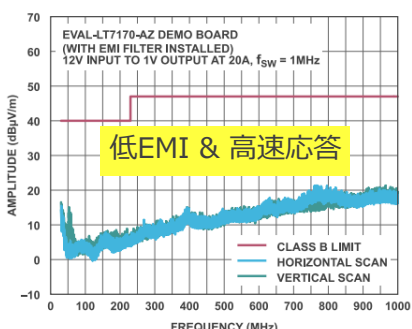
2相出力：LT7170-1
