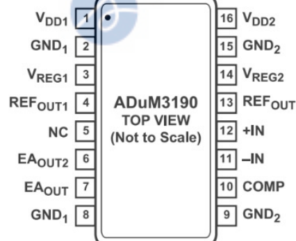
パッケージ(16pin QSOP)
