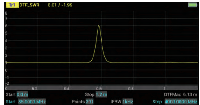
「VSWR vs. 距離」
