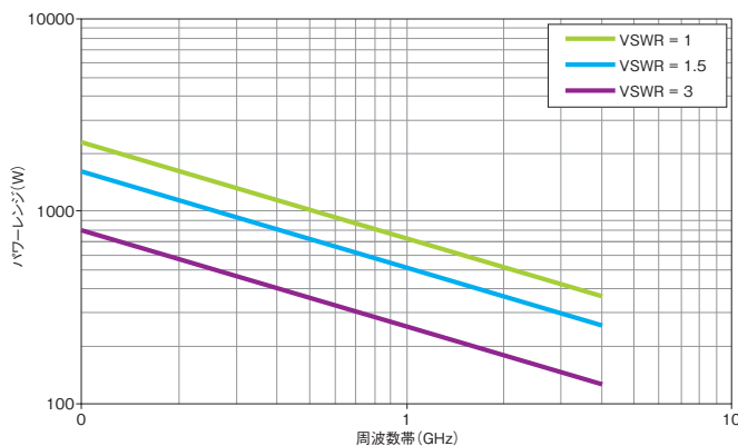
ピークパワー定格
