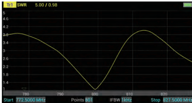
「VSWR vs. 周波数帯域」
