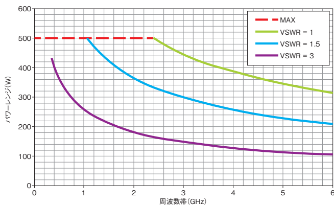
アベレージパワー定格
