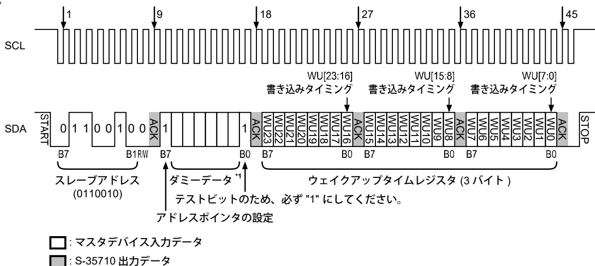
図24 ウェイクアップタイムレジスタの書き込みタイミング
