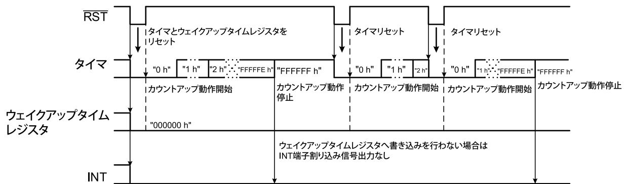
図15 ウェイクアップタイムレジスタに書き込みを行わない場合 (S-35710B01I / CMOS出力)
