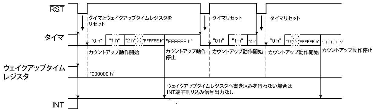
図14 ウェイクアップタイムレジスタに書き込みを行わない場合 (S-35710C01I / Nchオープンドレイン出力)
