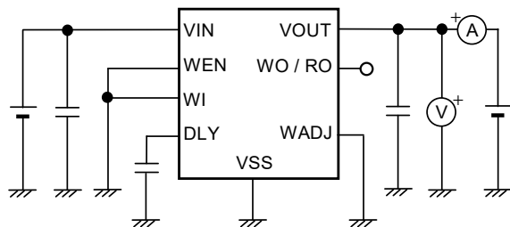
図11 測定回路2
