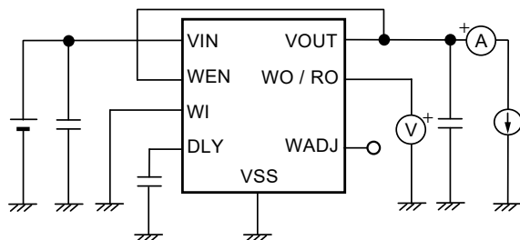
図15 測定回路6
