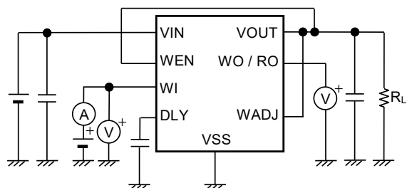
図17 測定回路8
