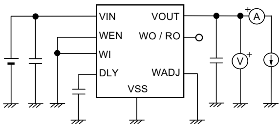
図10 測定回路1
