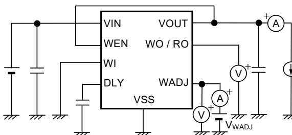
図16 測定回路7
