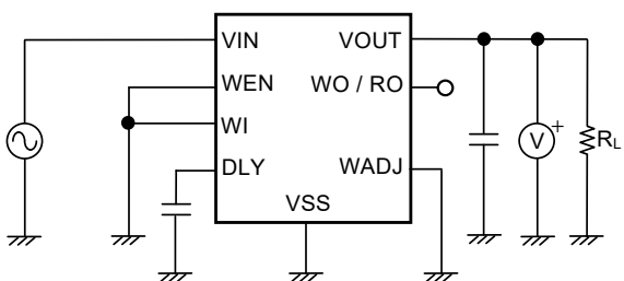
図12 測定回路3
