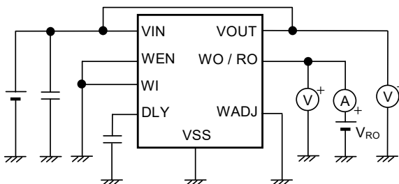
図14 測定回路5
