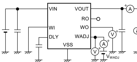
図26 測定回路7
