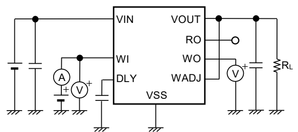
図27 測定回路8
