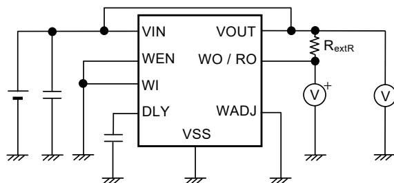
図13 測定回路4
