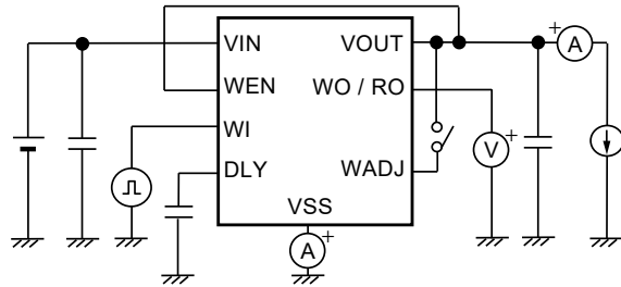
図19 測定回路10
