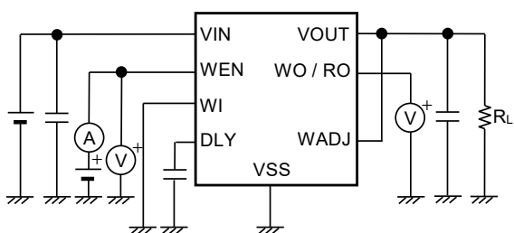
図20 測定回路9
