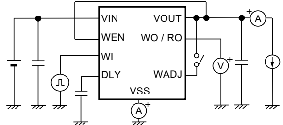
図21 測定回路10
