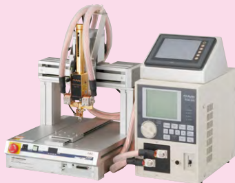
XYZ テーブル付き XYZ Table Type
